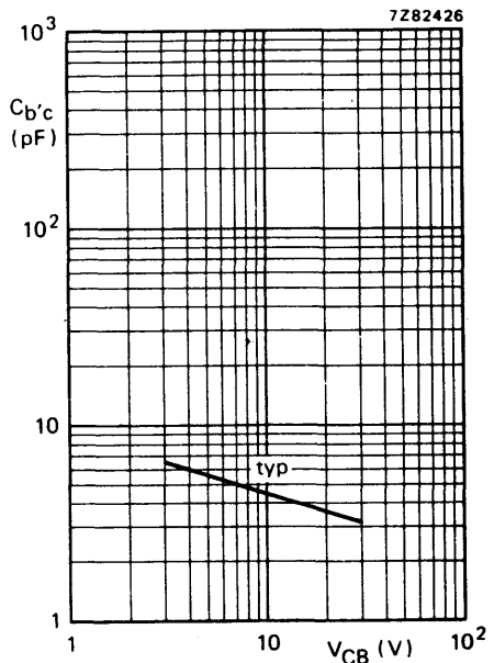
Fig. 12 f = 1\text{ MHz} ; T_{amb} = 25^\circ\text{C} .
