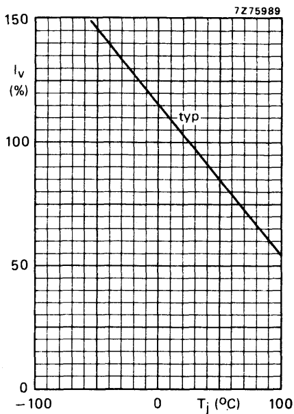
Fig. 10 I_F = 10\text{ mA} .
