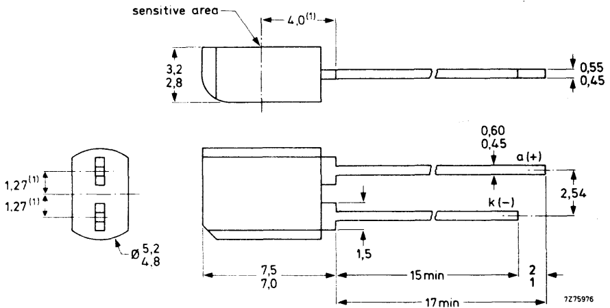
Fig. 1 SOD-67.
