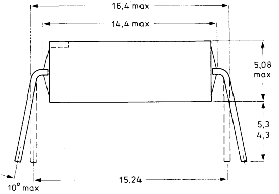
Fig. 1 SOT-91B.
