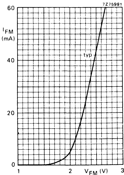
Fig. 7 t_p = 50 \mu\text{s} ; T = 5 \text{ ms} ; T_j = 25 \text{ °C} .
