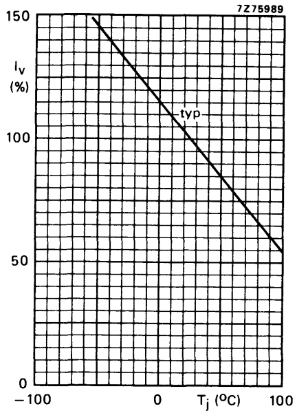
Fig. 10 I_F = 10 mA.
