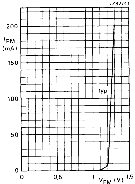
Fig. 6 T_{\text{amb}} = 25\text{ }^\circ\text{C} ; t_p = 10\text{ }\mu\text{s} ; T = 1\text{ ms} .
