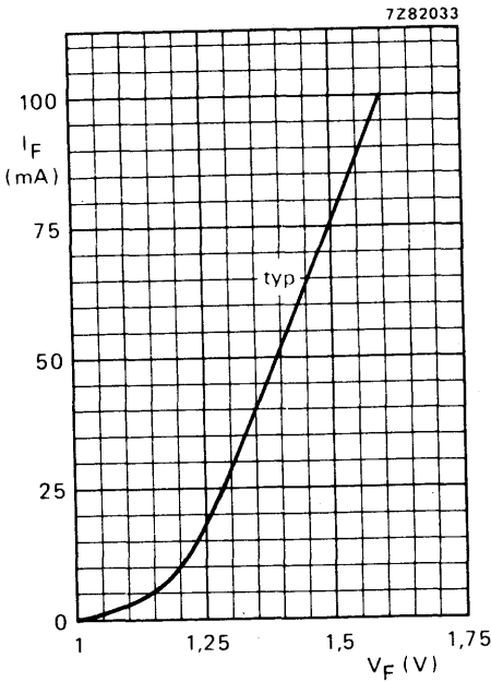
Fig. 5 T_{amb} = 25^\circ C .
