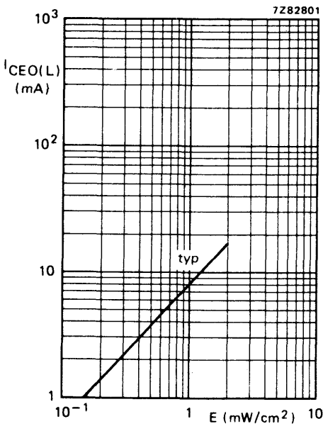
Fig. 8 V_{CE} = 5\text{ V} ; \lambda = 930\text{ nm} ; T_j = 25\text{ }^\circ\text{C} .
