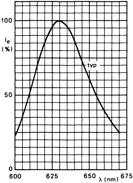
Fig. 8 CQW10.
