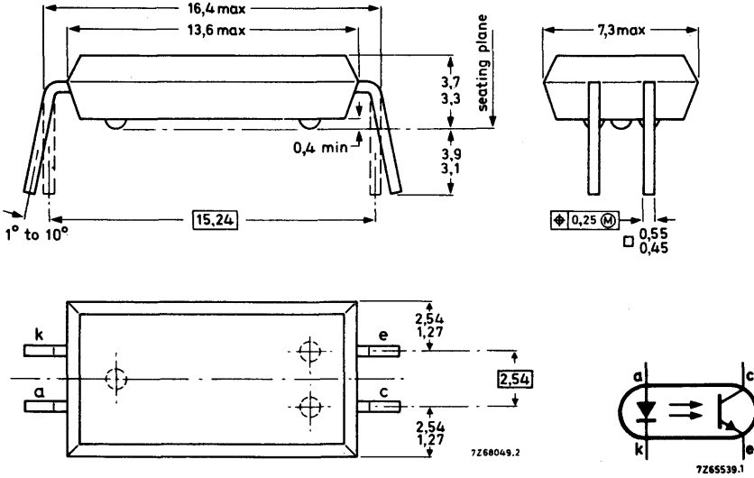
Fig. 1 SOT-91B.
