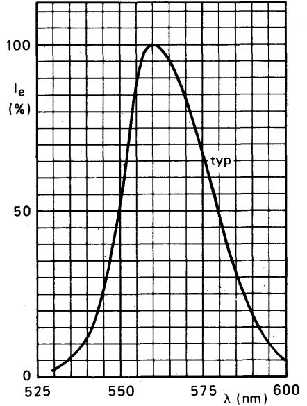
Fig. 9 CQW11.
